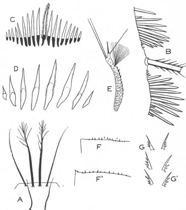
FIG. 5. — A, Anopheles nili Theobald, soies clypeales d'une larve ; B, Toxorhynchites viridibasis Edwards, partie distale de la selle de la larve ; C, Ficalbia circumtestacea Theobald, épines du 8 e segment abdominal de la larve, l'une d'elles étant représentée telle qu'on la voit à l'immersion ; D, Ficalbia uniformis Theobald, épines du 8 e segment de la larve, l'une d'elles étant représentée telle qu'on la voit à l'immersion ; E, Ficalbia circumtestacea Theobald, antenne de la larve ; F, F', G, G', Culex univittatus Theobald, partie distale de la selle de la larve (F et G = Sakaby, C, 140, 23-12-52 ; F' et G' = Dandé, B, 13-11-53) et épines les plus apicales du peigne du siphon.
