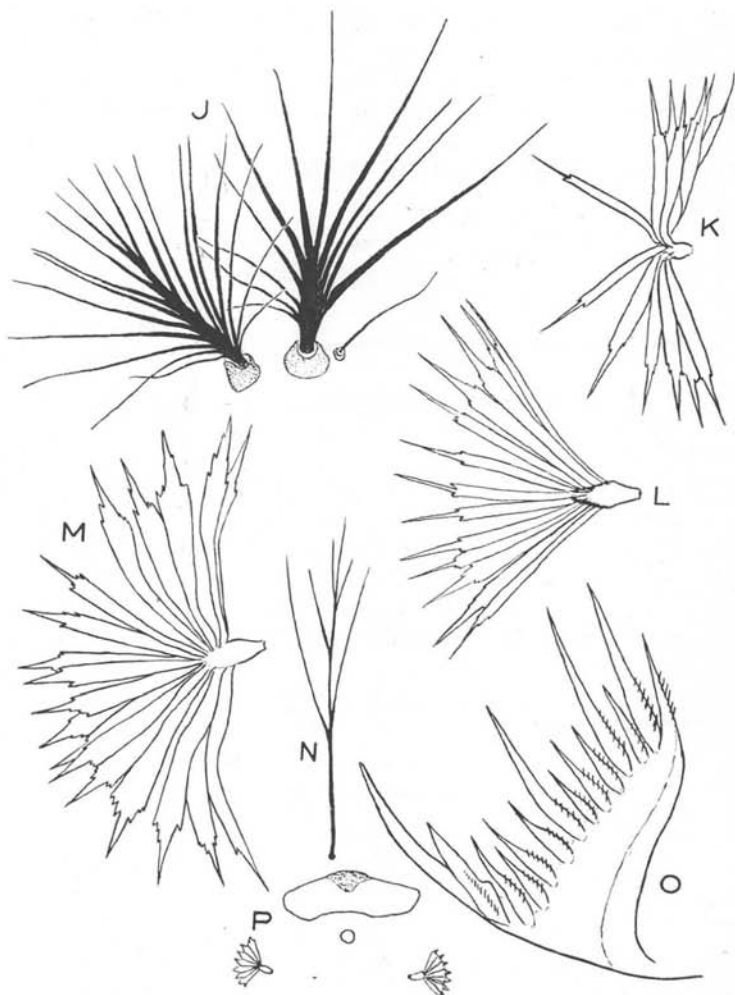
FIG. 2. — Anopheles hancocki var. masseguini nov. var. Larve : K, soies thoraciques submédianes droites; L, soie palmée thoracique; M, soie palmée du 1 er segment abdominal; N, soie palmée du 2 e segment abdominal; O, soie palmée du 5 e segment abdominal; P, plaques tergaux des segments abdominaux 4 à 6; Q, soie latérale de la selle; R, peigne du 8 e segment abdominal (les figures L, M, N, O sont à la même échelle).
